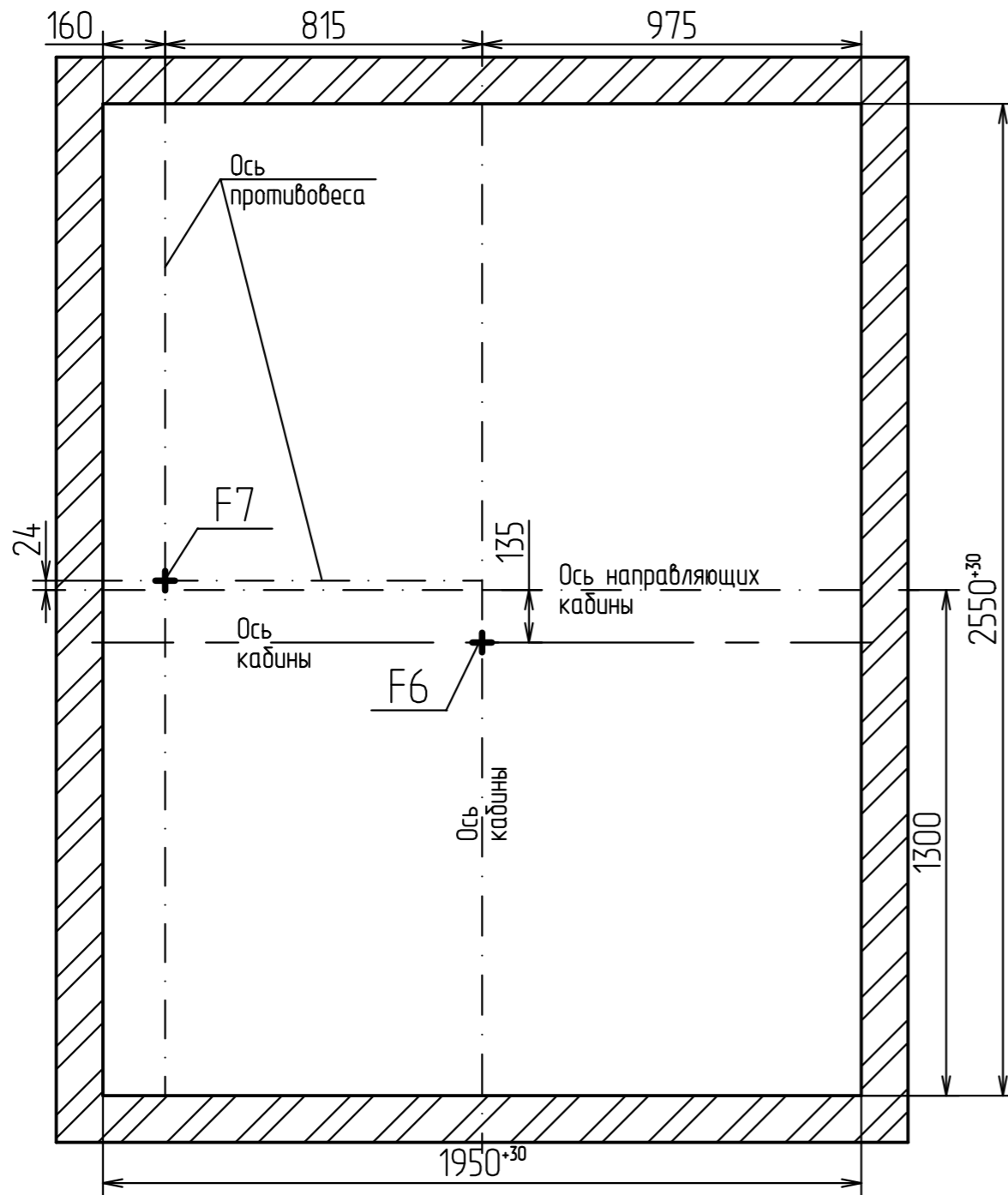
Г - Г (1) Схема приложения нагрузок на устройства для подвески грузоподъемных средств.
