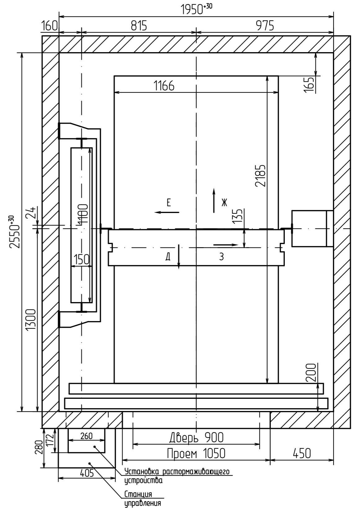
В - В (1) План шахты 1950 +30
